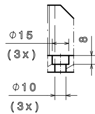
Section view A-A Scale: 1:2
